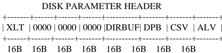
Figure 6-2. Disk Parameter Header Format
